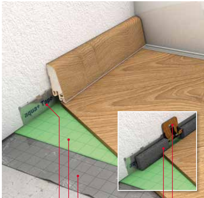
aqua + Alutape silenzio Easy aqua + Aluflex Nastro distanziatrice Clipstar
